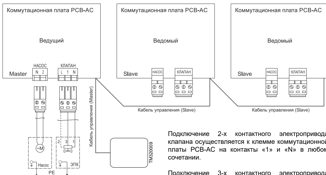
Схема подключения насоса и электропривода клапана к группе завес
